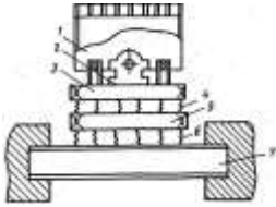
Рисунок 6 – Выбивная решетка [26]
