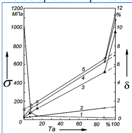
Рис. 7. Залежність механічних характеристик ШКМ Cu-Ta (без прошарків Ni) від об'ємного вмісту танталу: 1 - відносне подовження \delta ; 2 - теоретична границя пружності \sigma_{0,05} ; 3 - експериментальна границя пружності \sigma_{0,05} ; 4 - умовна границя текучості \sigma_{0,2} ; 5 - границя міцності \sigma_B
