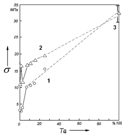
Рис. 8. Залежності \sigma_{0,05} і \sigma_B для ШКМ Cu-Ta з нікелевими прошарками від об'ємної долі Та: 1 - границя пружності \sigma_{0,05} ; 2 - границя міцності \sigma_B ; 3- дисперсія (розкид) апроксимованих значень \sigma_{0,05} і \sigma_B при 100% Та.
