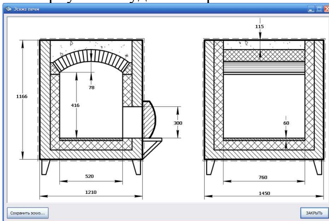
Рисунок 4 – Эскиз печи построенный программой
