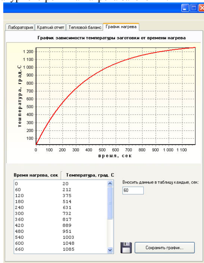
Рисунок 3 – График нагрева
