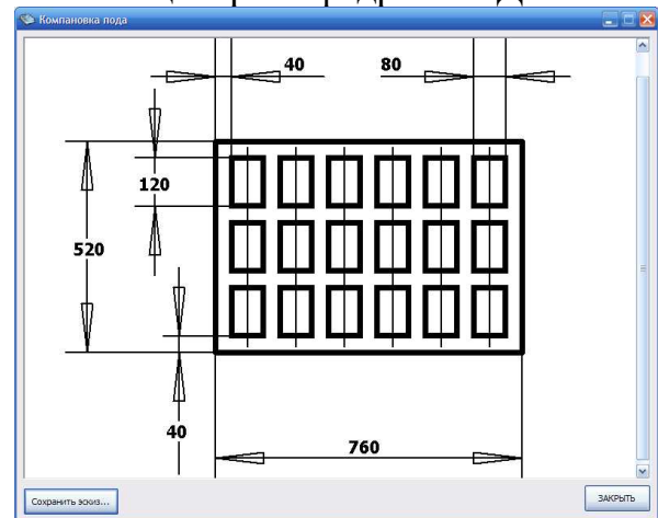
Рисунок 5 – Эскиз пода построенный программой
