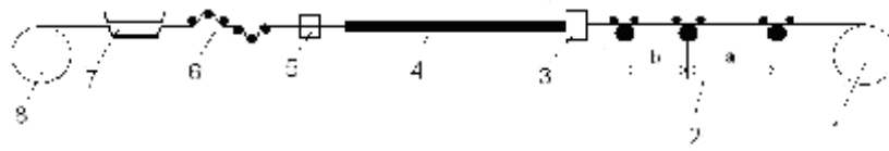
Рис. 1 Схема размещения агрегатов экспериментального участка подготовки металла к холодной деформации (обозначения в тексте)
