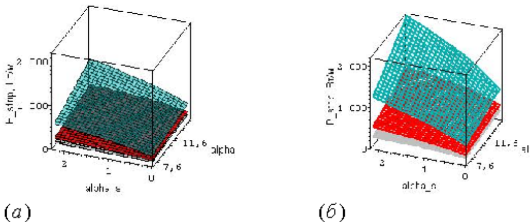
Рисунок 4 – Карти-поверхні прогнозованої погонної потужності БЕТСО для режимів I, III і V при термостабілізації поверхні підлоги на рівнях нагріву t_{зд} = (a) 18C^{\circ}; (б) 38C^{\circ} при зміні параметрів теплообміну a і a_g
