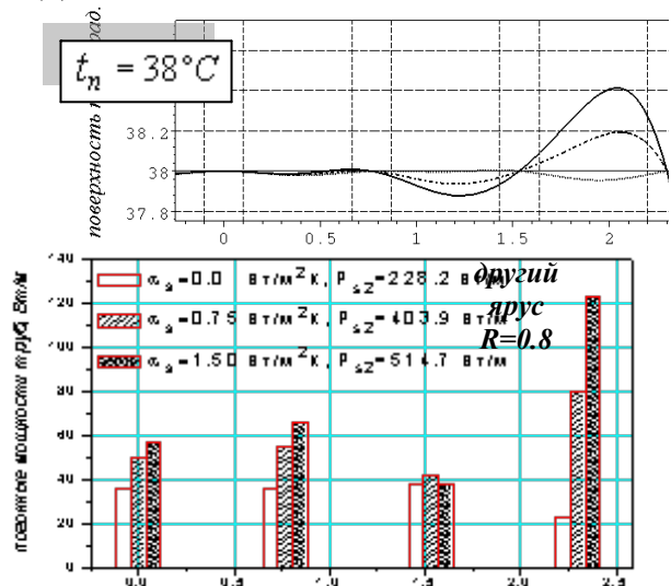
Рисунок 2 – Розподіл температури на поверхні підлоги та відповідні енергограми НС для режиму II при R=0.8 (а), R=0.6 (б) та R=0.4 (в)
