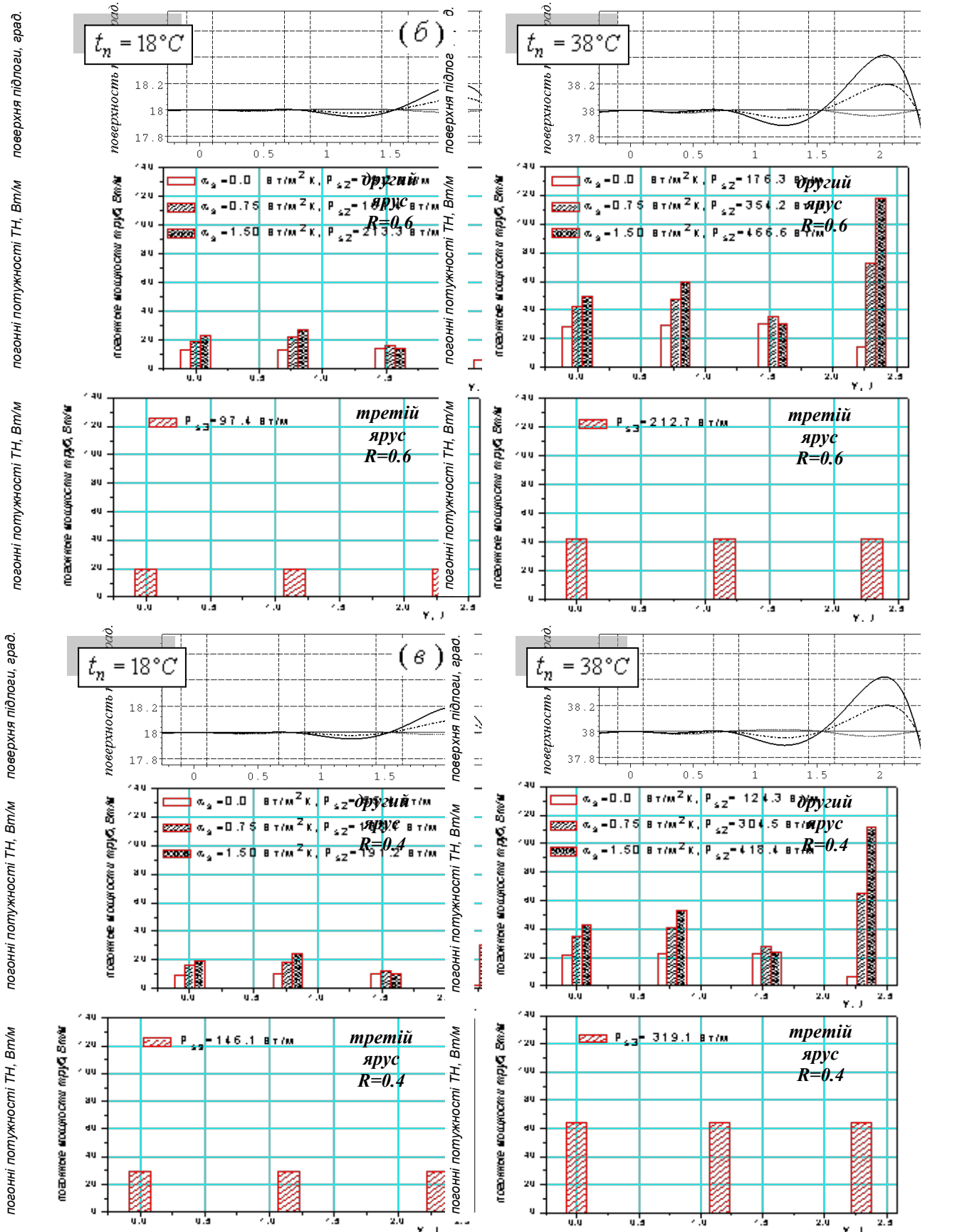
Рисунок 3 – Розподіл температури на поверхні підлоги та відповідні енергограми НС для режиму IV при R=0.8 (а), R=0.6 (б) та R=0.4 (в)
