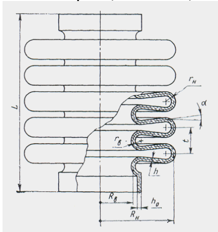
Рис. 1. Схема сильфона
