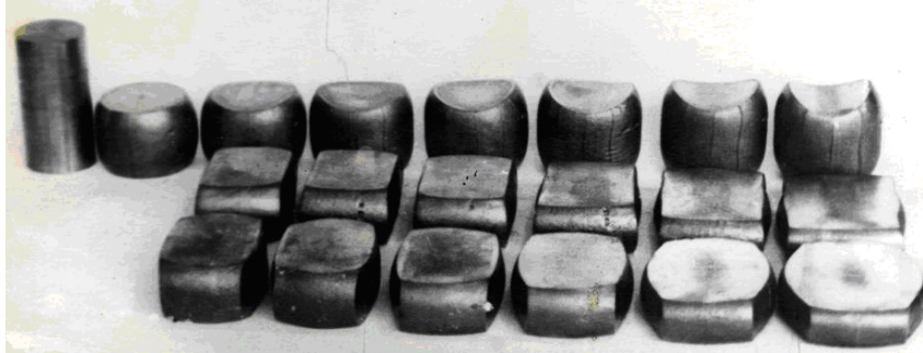
Рис. 8. Заготовки, осаженные выпуклыми продолговатыми плитами различной радиусности и разглаженные по различным схемам
