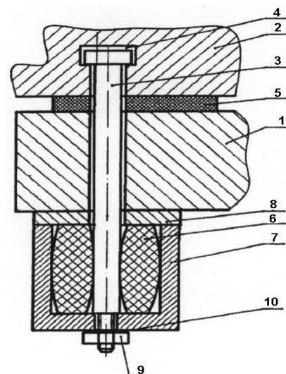
Рис. 3. Узел крепления верхней плиты штампа к ползуну пресса: 1 – верхняя плита; 2 – ползун; 3 – стяжной винт; 4 – паз; 5 – пластина компенсатора; 6 – упругий элемент; 7 – втулка или стакан; 8 – шайба; 9 – гайка; 10 – пружинная шайба
