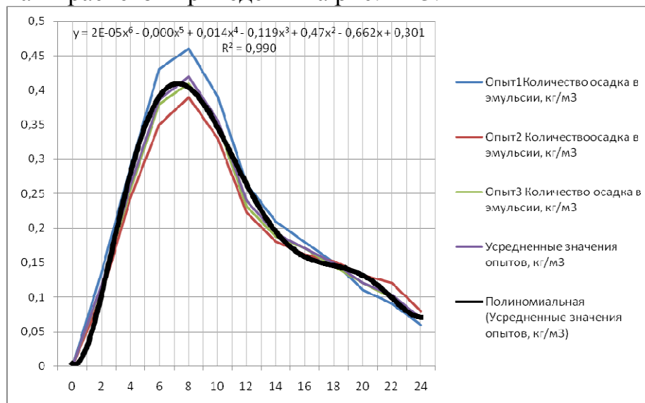
Рис.2. Результаты эксперимента по осаждению механических примесей в промышленных условиях.
