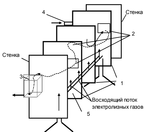
Рис.4 Схема перегородок в аппарате фракционированного коагулирования 1 - перегородки; 2 – потоко - направляющие отверстия; 3 - карман отвода очищенной воды; 4 - патрубок подачи воды на очистку; 5 - щелевидный канал.
