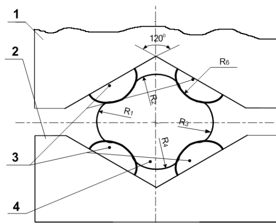
Рис.2. Обжатие заготовки вырезными профилированными бойками 1- боёк вырезной верхней; 2 - боёк вырезной нижней; 3 - четыре выпуклые вставки; 4-заготовка
