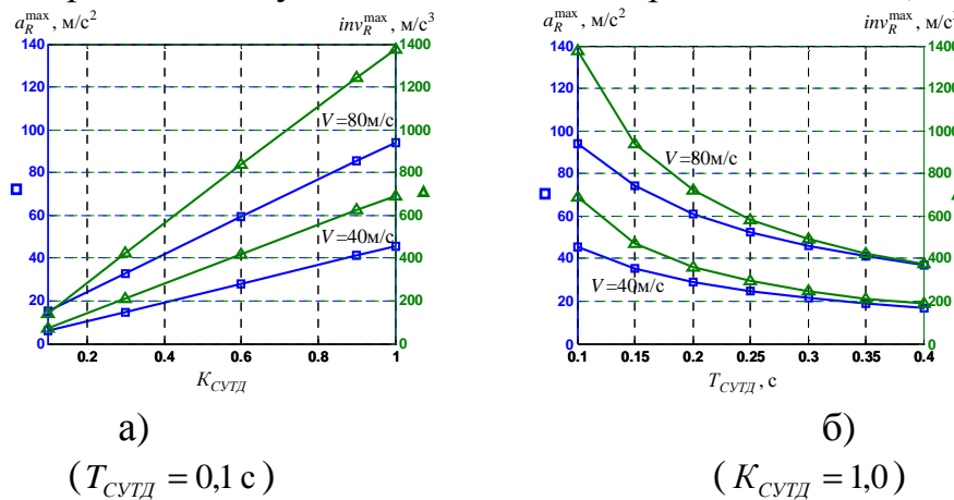
Рис. 5. Зависимость максимальных значений высших производных дальности от параметров системы управления тягой двигателя
