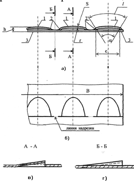
Рис. 4 - Надрезанная лента дугообразным ножом (фронтальный вид)
