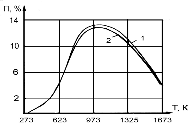
Рис. 2 Зміна відкритої пористості покриття на основі наповненого \text{Al}_2\text{O}_3 і \text{ZrO}_2 поліалюмосилоксану (1) та з додатком 5 мас.% каолінового волокна (2)
