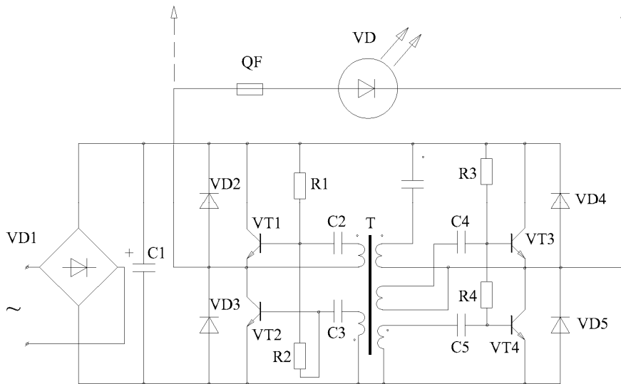
Рис.2. Принципова електрична схема блока живлення СД-модуля
