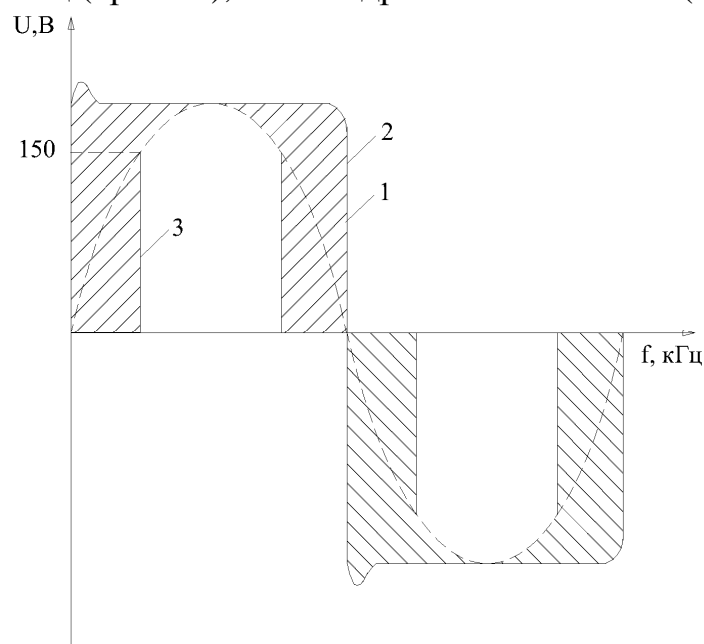
Рис.1. Осцилограми роботи СД-модуля “Acriche”.
