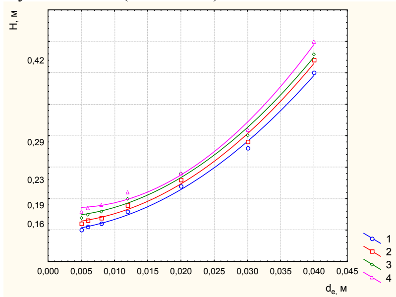
Малюнок 2. – Залежність висоти піни від діаметру отворів решітки: 1 - w_2 = 3 м/с, L_0 = 7 м 3 /м 2 год, 2 - w_2 = 3 м/с, L_0 = 10 м 3 /м 2 год, 3 - w_2 = 4 м/с, L_0 = 7 м 3 /м 2 год, 4 - w_2 = 4 м/с, L_0 = 10 м 3 /м 2 год.
