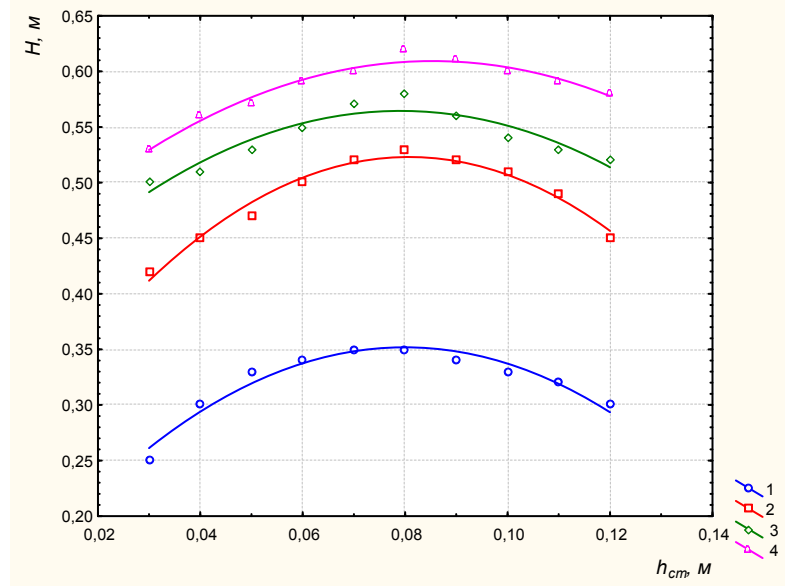
Малюнок 4. – Залежність висоти пінного шару від розташування насадки над полотном тарілки: S_0 = 0,33 \text{ м}^2/\text{м}^2 ; d_e = 0,04 \text{ м} , L_0 = 2 \text{ м}^3/\text{м}^2\text{год} ; w_2 : 1 - 2 м/с, 2- 2,5 м/с, 3 – 3 м/с, 4 – 3,5 м/с.
