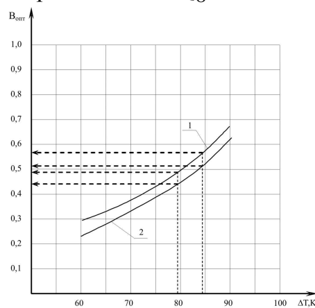
Рис. 9. Зависимость величины \frac{\lambda_{\Sigma}}{n_1 \lambda_0} двухкаскадного ТЭУ от отношения количества термоэлементов в смежных каскадах \frac{n_1}{n_2} и от перепада температур \Delta T при T = 300 \text{ K} , Q_0 = 0,1 \text{ Вт}
