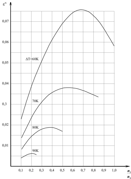
Рис. 8. Зависимость холодильного коэффициента \epsilon^N двухкаскадного ТЭУ от отношения количества термоэлементов в смежных каскадах \frac{n_1}{n_2} при T = 300 \text{ K} , Q_0 = 0,1 \text{ Вт} и перепадах температур \Delta T = 60 \text{ K} ; 70 \text{ K} ; 80 \text{ K} ; 90 \text{ K}
