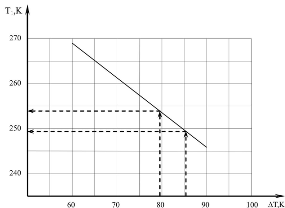
Рис. 12. Зависимость промежуточной температуры T_1 , обеспечивающей наименьшую интенсивность отказов двухкаскадного ТЭУ, от перепада температур \Delta T при T = 300 К, Q_0 = 0,1 Вт
