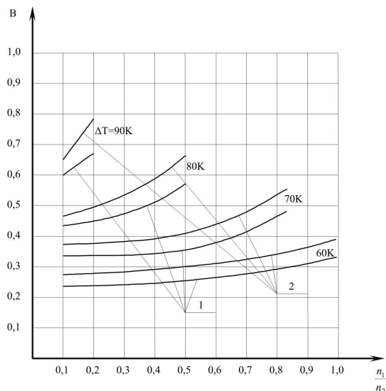
Рис.1 Зависимость относительного рабочего тока в каскадах B_1 и B_2 двухкаскадного ТЭУ от отношения количества термоэлементов в
