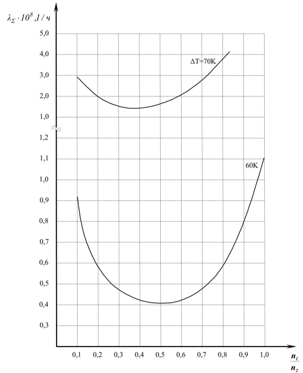
Рис. 5. Зависимость интенсивности отказов \lambda_{\Sigma} двухкаскадного ТЭУ от отношения количества термоэлементов в смежных каскадах \frac{n_1}{n_2} при n_1 = 9 , T = 300 \text{ K} , Q_0 = 0,1 \text{ Вт} и перепадах температур \Delta T = 60 \text{ K} ; 70 \text{ K} .
