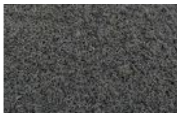
Рис.3. Аморфный осадок, выделяющийся на стенках реактора при соотношении \text{SiCl}_4:\text{C}_7\text{H}_8=3,5 (x 750)
