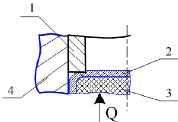
Рис. 1. Схема разделения металла классическим способом при пробивке эластичной средой, начало процесса:
