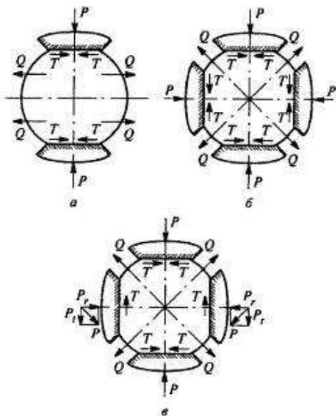
Рис. 3. Ковка слитков на прессе двумя бойками (а), на РКМ (б) и четырехбойковом устройстве (в). Р – действующие силы; Q – потоки вытеснения металла; T – силы трения
