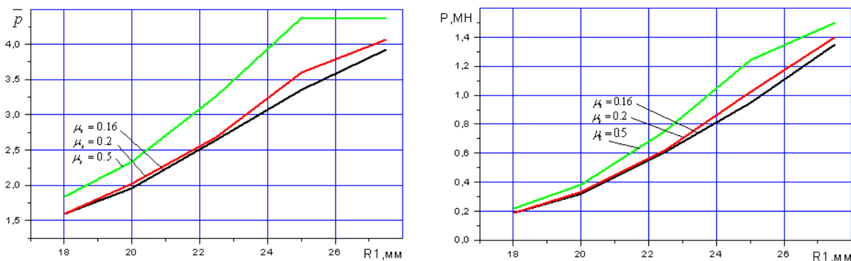
Рис. 5. Графики зависимости приведенного давления и усилия деформирования от радиуса матрицы (QForm)
