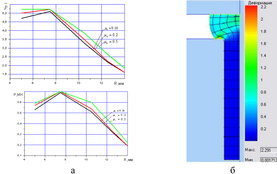
Рис. 4. Графики зависимости приведенного давления и усилия деформирования от радиуса оправки (QForm):
