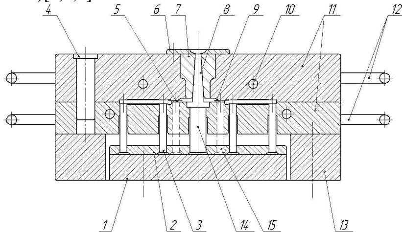
Рис. 8. Схема пресс формы литья под давлением .
