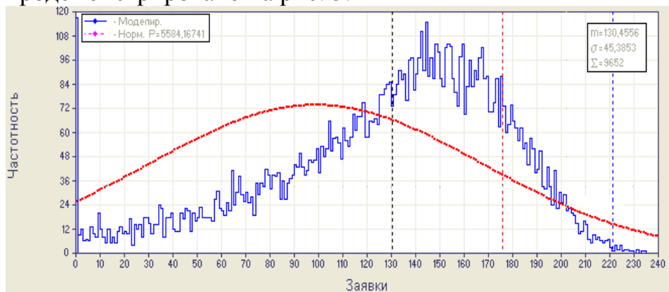
Рис. 3. Распределение количества заявок за интервал времени
