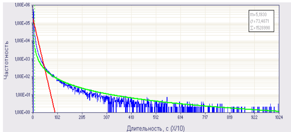
Рис. 2. Аппроксимация интервала времени между заявками
