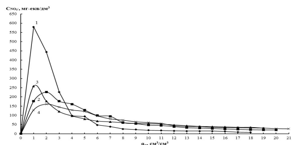
Рис. 3. Вплив питомої витрати розчинів хлориду натрію (10 %) (1), сульфату натрію (10 %) (2), луку (4 %) (3) та соди (10 %) (4) при пропусканні через високоосновний аніоніт АВ-17-8 в NO_3^- -формі на зміну концентрації нітратів в вихідному розчині
