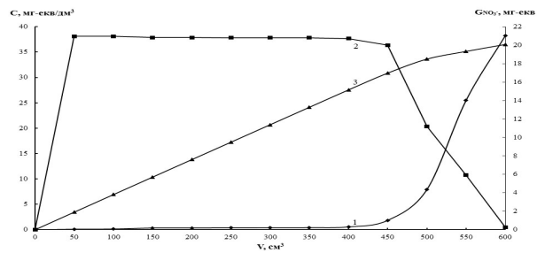
Рис. 2. Залежність концентрації нітратів (1), хлоридів (2) та кількості сорбованих нітратів (3) від пропущеного об'єму розчину нітрату натрію ( C_{NO_3^-} = 38,226 \text{ мг-екв/дм}^3 = 2370 \text{ мг/дм}^3 ) через аніоніт АВ-17-8 в СІ-формі ( V_i = 10 \text{ см}^3 ) ( ПОДЕ_{NO_3^-} = 2010 \text{ мг-екв/дм}^3 )
