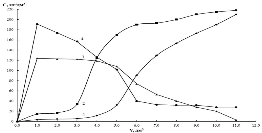
Рис. 6. Залежність концентрації нітратів (1, 2) та хлоридів (3, 4) від об'єму пропущеного розчину нітрату натрію у дистильованій воді ( C_{\text{NO}_3^-}=220 мг/дм 3 ) (1, 3) та у водопровідній воді ( C_{\text{NO}_3^-}=250 мг/дм 3 , C_{\text{Cl}^-}=28 мг/дм 3 , C_{\text{SO}_4^{2-}}=38 мг/дм 3 ) через низькоосновний аніоніт DOWEX Marathon в \text{Cl}^- -формі ( V_i=20 см 3 ) (ПОДЕ 1 NO 3 - =1184 мг-екв/дм 3 ; ПОДЕ 2 NO 3 - =873 мг-екв/дм 3 )
