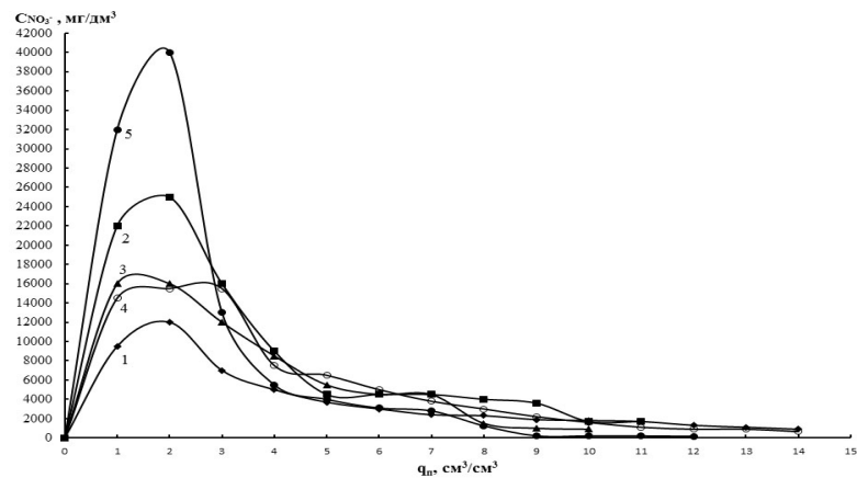
Рис. 7. Вплив питомої витрати ( q_{п} ) 10 %-них розчинів NaCl (1), NH 4 Cl (2), KCl (3), K 2 CO 3 (4) та 4 %-ного розчину NH 4 OH (5) на концентрацію нітратів в цих розчинах при пропусканні їх через низькоосновний аніоніт DOWEX Marathon в NO 3 - -формі
