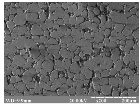
Рис. 2 Мікроструктура брукту системи W-Ni-Fe
