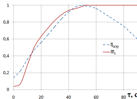
Рис.3 \bar{q}_{aэp} – изменение относительного количества паров кислорода в свободном объеме бака при работе системы наддува по времени полета: \bar{m}_s = m_{si} / m_{smax} – масса паров кислорода на i -тый момент времени; \bar{q}_{aэp} = q_{aэpi} / q_{aэpmax} – номинальный аэродинамический тепловой поток в стенку бака окислителя на i -тый момент времени
