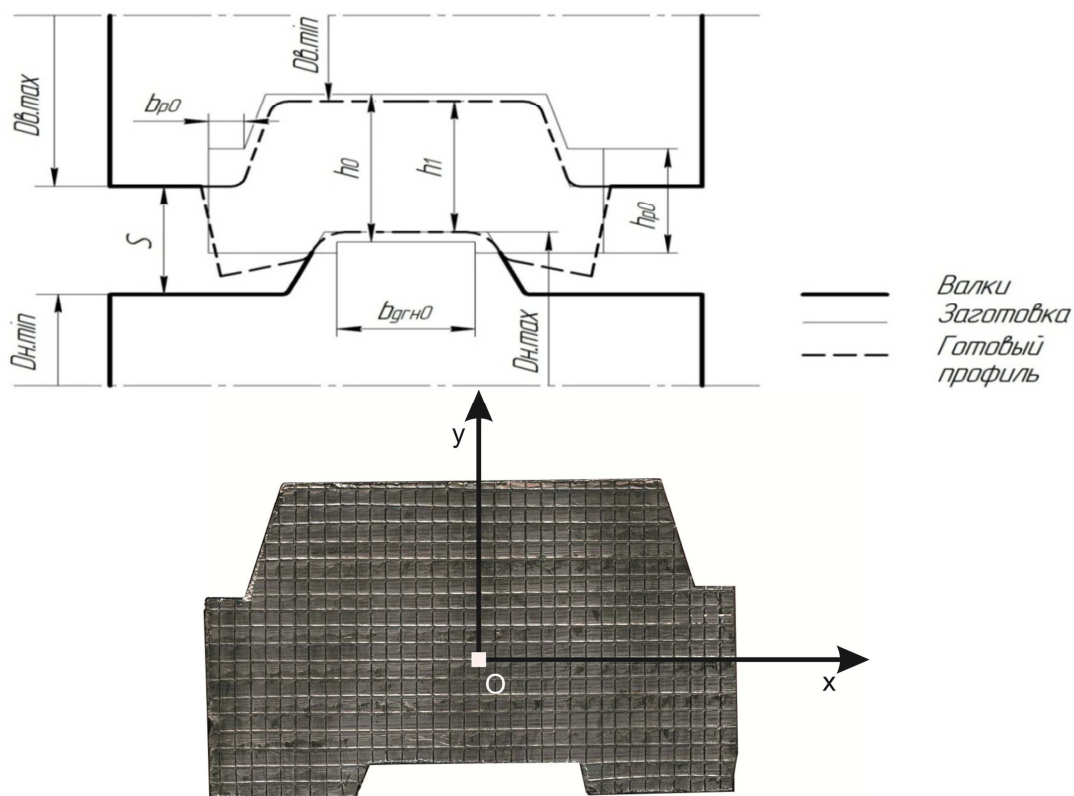
Рис. 1 – Схема деформации и заготовка с нанесенной сеткой
