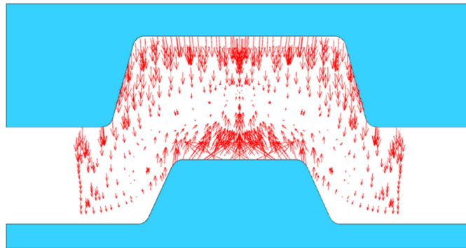
Рис. 3 – Поле скоростей в векторном виде
