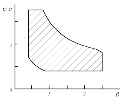
Рис. 2. Диапазон изменения условных показателей \beta = \sqrt{S_{эл}} / 2t и b/a электромагнитов (уточнённые данные для коэрцитиметра КРМ-Ц)
