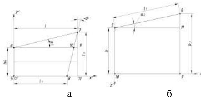
Рис. 2 - Ескізи проекцій моделі ДБ НА: а- фронтальна проекція; б- ескіз в плані
