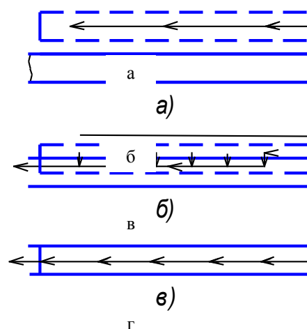
Рис.2 - Схема течії матеріалу в каналах ротора і корпусу: 1 – вхідне поглиблення ротора; 2 – вихідне поглиблення корпусу: а – поглиблення не сполучаються; б – сполучаються частково; в – сполучаються повністю; г – поглиблення вийшли з сполучення
