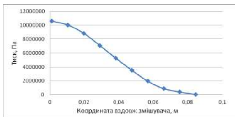
Рис. 5 - Графік розподілу тиску по довжині каналу змішувача
