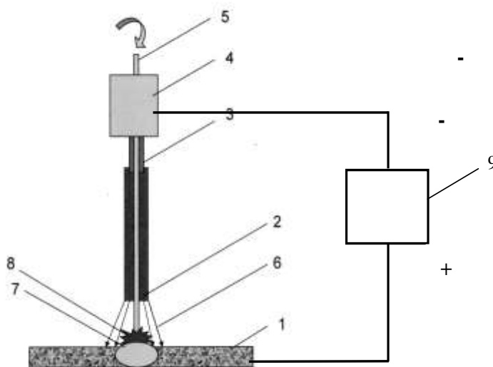
Рис.1 - Схема виконання способу зварювання чавуну
