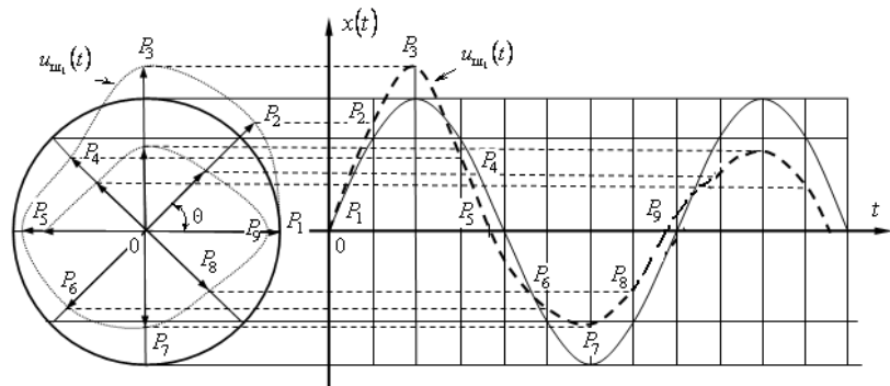
Рис. 1 - Процесс формирования хаотического сигнала x_{sc}(t) на основе синусоидального колебания
