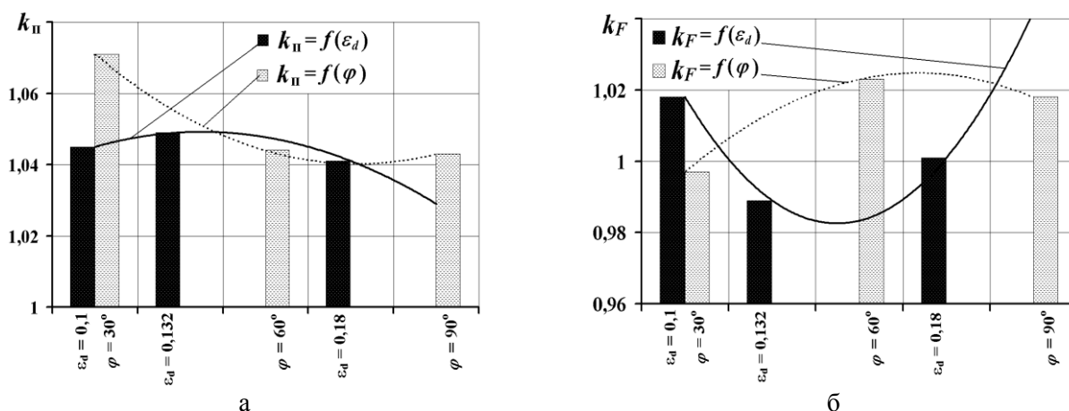
Рис. 9 – Результаты исследования геометрических характеристик поперечного сечения образцов при различных режимах обжатий в комбинированных бойках: с использованием коэффициентов:
