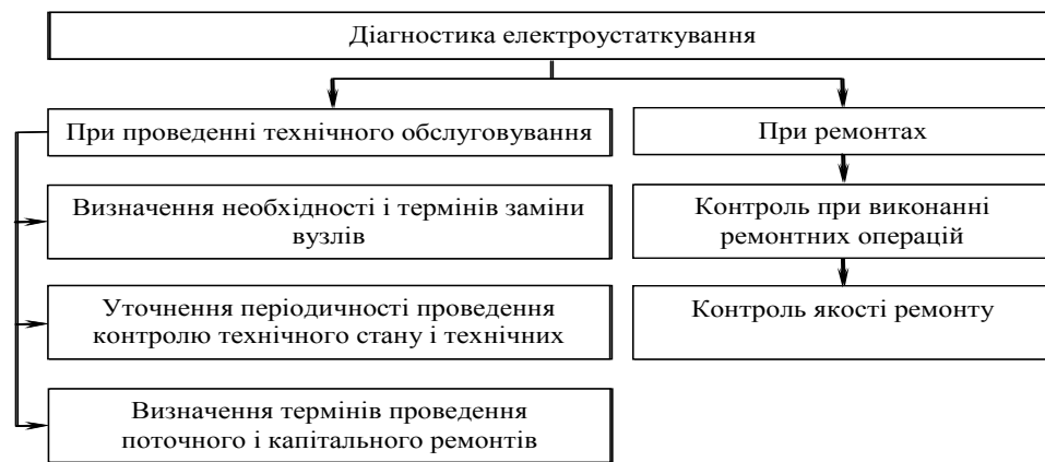
Рис. 2 – Область застосування технічних засобів діагностики при використанні ОФС
