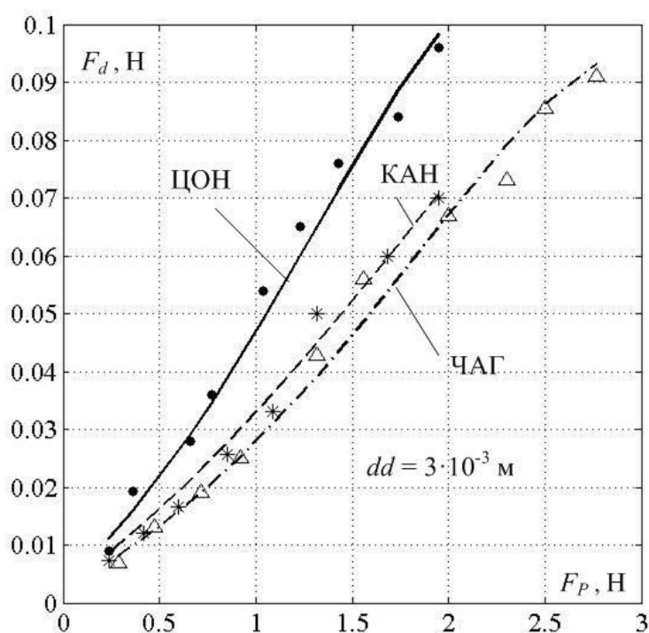
Рис. 6 – Залежність експериментальних і розрахованих значень F_d від притискання перетворювача F_P
