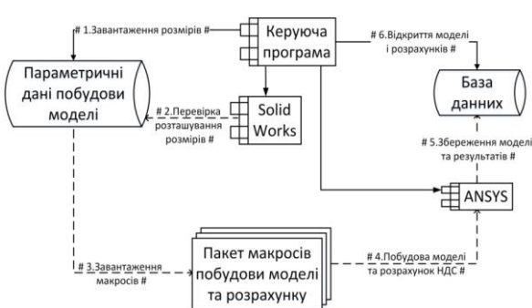
Рис. 10 – Діаграма компонентів
