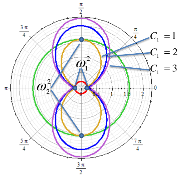
Рис. 3 – Изменение характерного сечения в плоскости \omega_1, \omega_2 3х мерной фигуры при варьировании жесткости i й пружины
