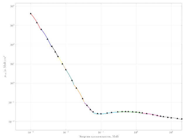
Рис. 1 – Зависимость массового коэффициента ослабления для воды от энергии гамма кванта. ▲ - табличные данные зависимости коэффициента массового ослабления для воды.
