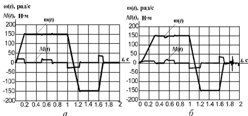
Рис. 2 Переходные процессы в бездатчиковом электроприводе при: а) номинальных параметрах двигателя; б) увеличении активного сопротивления ротора АД на 20%
