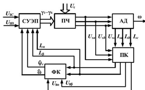
Рис. 1 Структура бездатчикового векторного асинхронного электропривода
