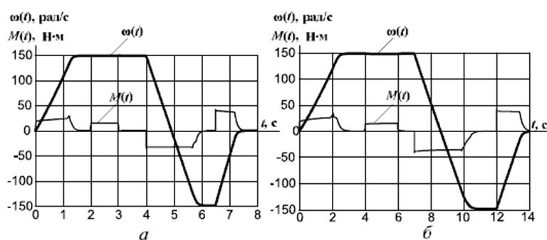
Рис. 6 Переходные процессы в бездатчиковом электроприводе при увеличении момента инерции АД в: а) 10; б) 20 раз
