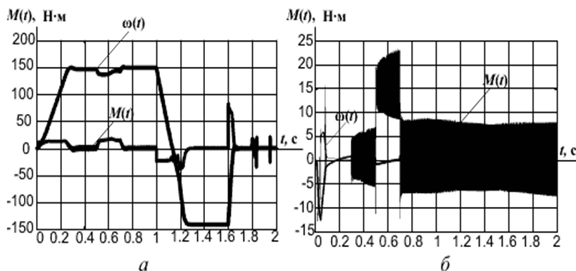
Рис. 3 Переходные процессы в бездатчиковом электроприводе при увеличении активного сопротивления ротора АД на: а) 35; б) 40%
