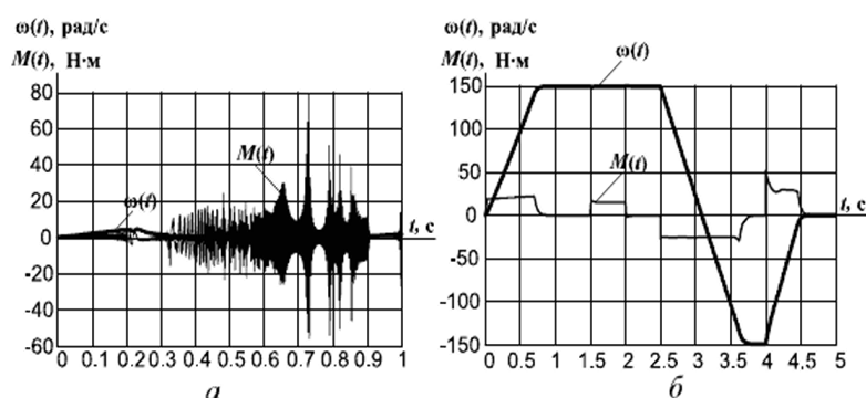
Рис. 5 Переходные процессы в бездатчиковом электроприводе при увеличении: а) индуктивности намагничивания АД на 70 %; б) момента инерции АД в 5 раз
