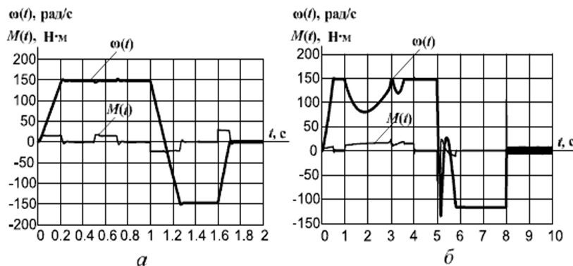
Рис. 4 Переходные процессы в бездатчиковом электроприводе при увеличении индуктивности намагничивания АД на: а) 25; б) 50 %
