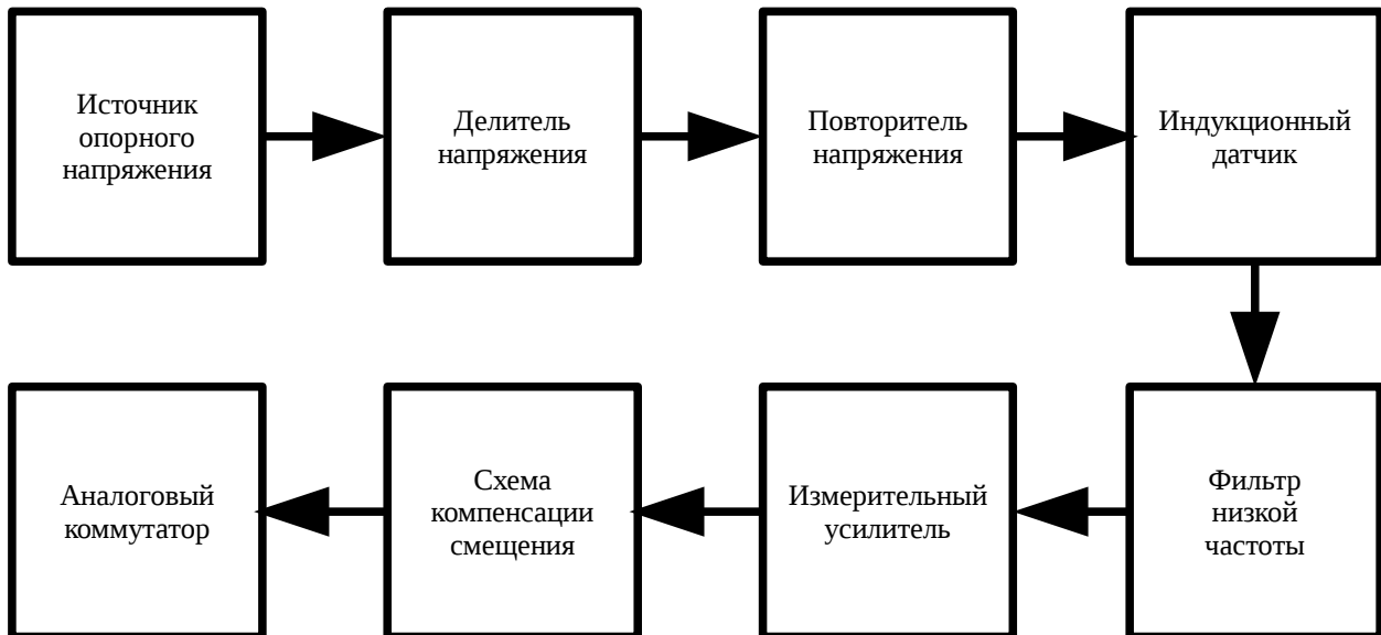
Рис. 1. – Структурная схема.
