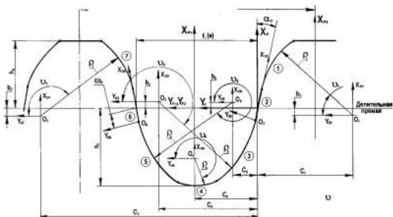
Рис. 1. Обобщенный исходный контур
