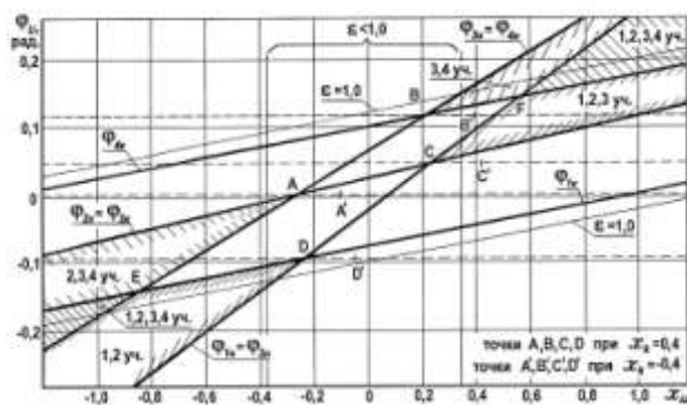
Рис.2. Диаграмма углов входа и выхода из зацепления по различным участкам.
