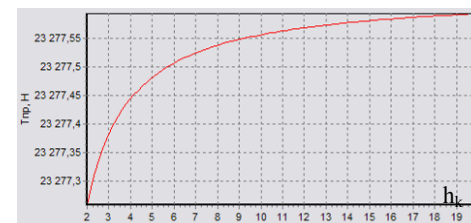
Рисунок 3 – Зависимость предельного вращающего момента от толщины жесткого колеса при i=80; E=2,1 \cdot 10^5 \text{ Н/мм}^2; G=8 \cdot 10^4 \text{ Н/мм}^2; D_{п}=120 \text{ мм}; L=500 \text{ мм}; h_d=3 \text{ мм} ; шариковый подшипник с Z_{ш}=20 и D_{ш}=6 \text{ мм}
