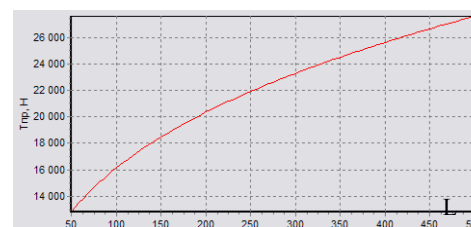
Рисунок 4 – Зависимость предельного вращающего момента от длины гибкого колеса при i=80; E=2,1 \cdot 10^5 \text{ Н/мм}^2; G=8 \cdot 10^4 \text{ Н/мм}^2; D_{п}=120 \text{ мм}; h_d=3 \text{ мм}; h_k=25 \text{ мм} ; шариковый подшипник с Z_{ш}=20 и D_{ш}=6 \text{ мм}
