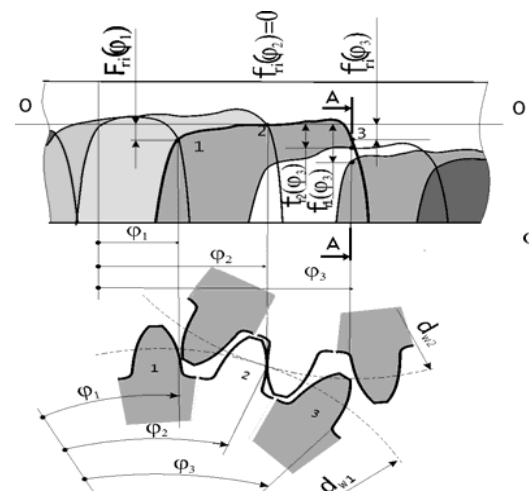
Рисунок 3 – Модель учета кинематического состояния зубьев в зацеплении
