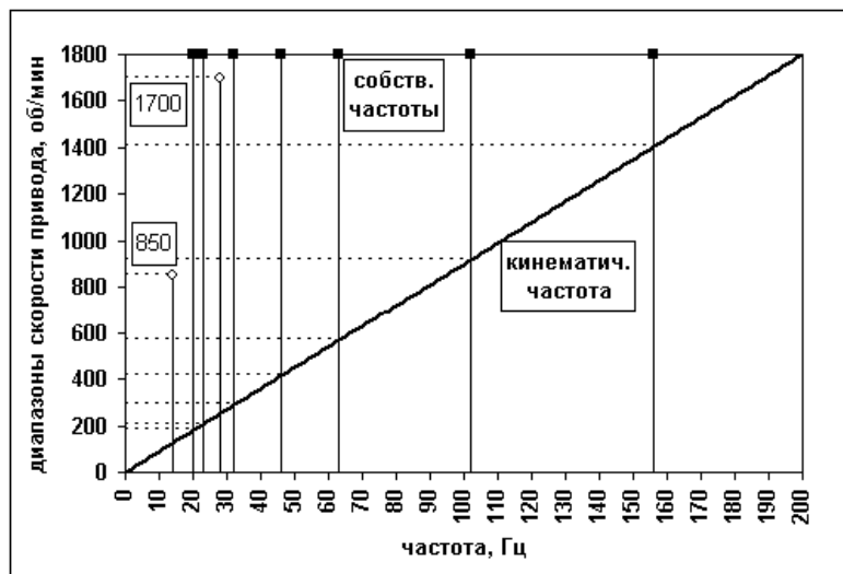
Рисунок 5 – Диаграмма кинематических и собственных частот РКБ
