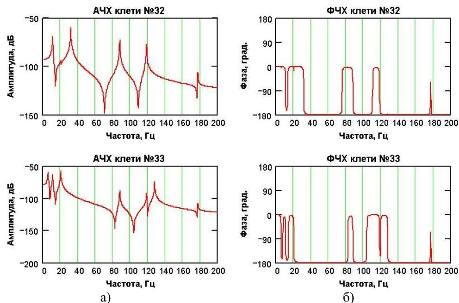
Рисунок 4 – АЧХ (а) и ФЧХ (б) клеток 32 и 33 РКБ
