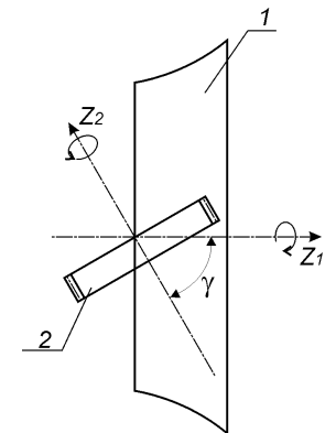
Рисунок 8 – Схема формообразования квазиглобоидной заготовки и квазиглобоидного червяка (колеса)
