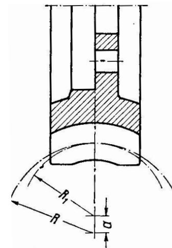
Рисунок 2 – Схема смещения оси червячной фрезы после переточки для получения нормальной высоты зуба червячного колеса
