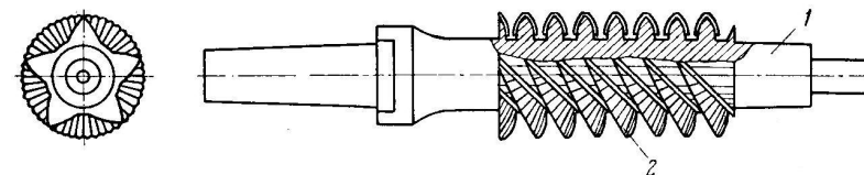
Рисунок 6 – Червячная фреза "Дэвид Браун"
