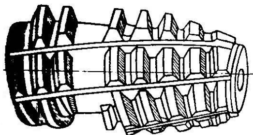
Рисунок 3 – Комбинированная червячная фреза
