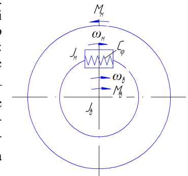
Рисунок 2 – Динамічна розрахункова схема
