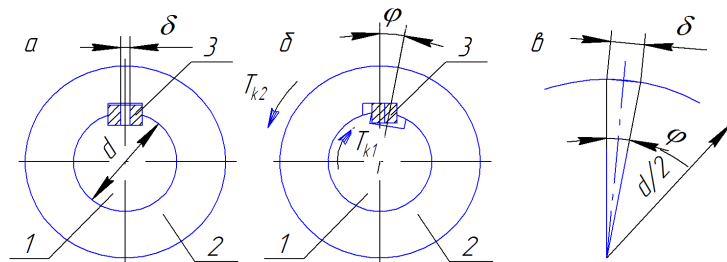
Рисунок 1 – Схеми роботи з'єднання типу "вал-маточина" з пружною призматичною шпонкою: а – до навантаження; б – після навантаження; в – для визначення кута повороту вала відносно маточини
