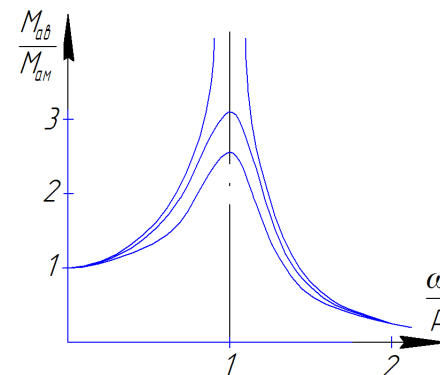
Рисунок 4 – Резонансна крива
