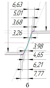
Рисунок 3 – Координаты опорных и управляющих точек сплайна
