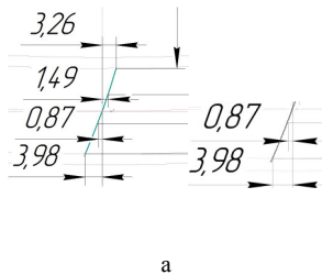
Рисунок 3 – Координаты опорных и управляющих точек сплайна
