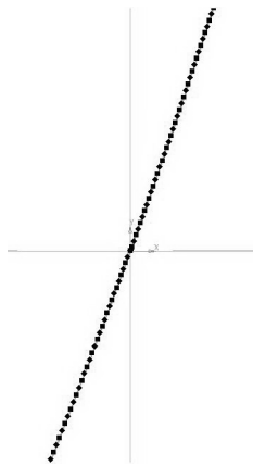
Рисунок 1 – Точки контура
