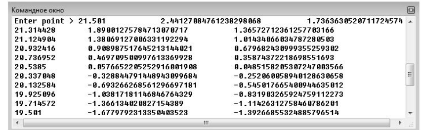
Рисунок 6 – Командное окно
