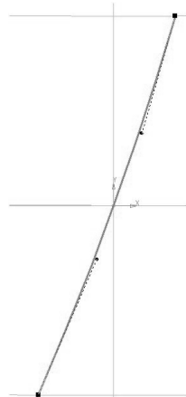
Рисунок 2 – Аппроксимация сплайном
