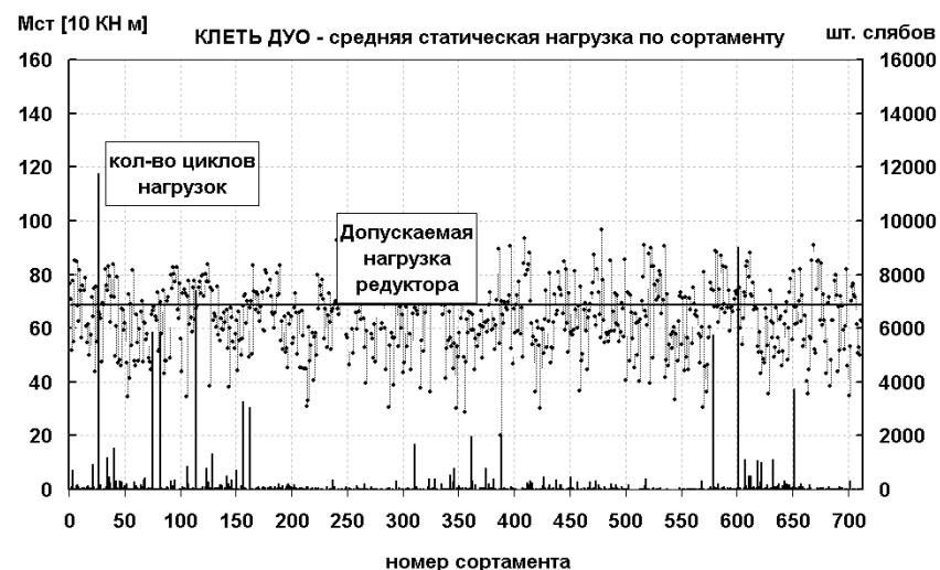
Рисунок 4 – Средняя по слябам статическая нагрузка в клетке дуо стана 1680
