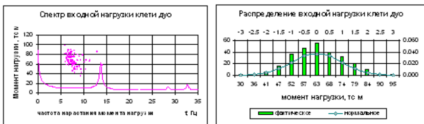
Рисунок 5 – Спектр технологической нагрузки в клети дуо стана 1680: а) спектр входной нагрузки и расчетный график АЧХ линии привода; б) стандартное распределение входной нагрузки
