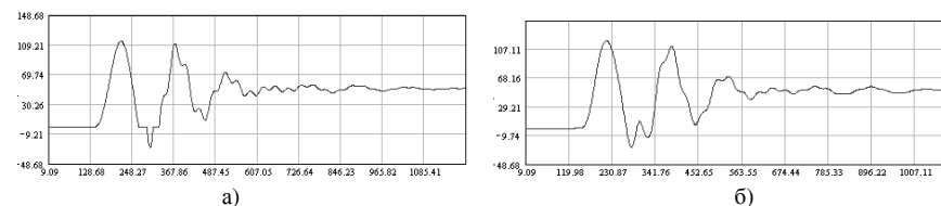
Рисунок 9 – Расчетные моменты сил упругости при раскрытии зазоров: а) в муфтах на моторном валу; б) в зацеплении входной ступени редуктора
