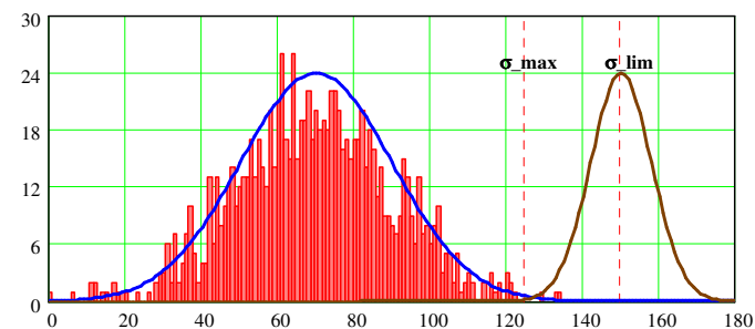
Рисунок 2 – График распределений максимальных значений момента сил упругости: \sigma_{max} – максимальная нагрузка ( 3\sigma ); \sigma_{lim} – средняя допустимая нагрузка
