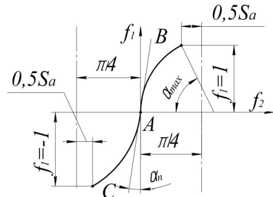
Рисунок 2 – Параметры исходного контура ( \alpha_n = 9,34^\circ ; \alpha_{\max} = 30,7^\circ ; 0,5S_a = 0,312 )
