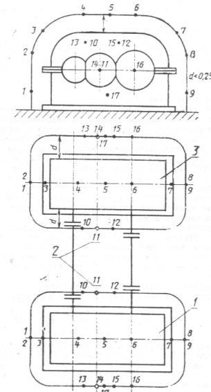
Рисунок 1 – Схема розміщень вимірювальних точок по методу [1]
