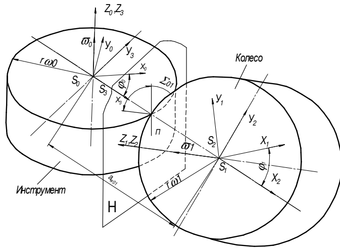
Рисунок – Схема станочного зацепления для нарезания шевера с неэвольвентной производящей поверхностью
