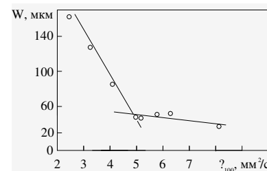
Рисунок 5 – Влияние вязкости v_{100} вазелинового масла с 1% диалкилдифосфата цинка на износ W [68]
